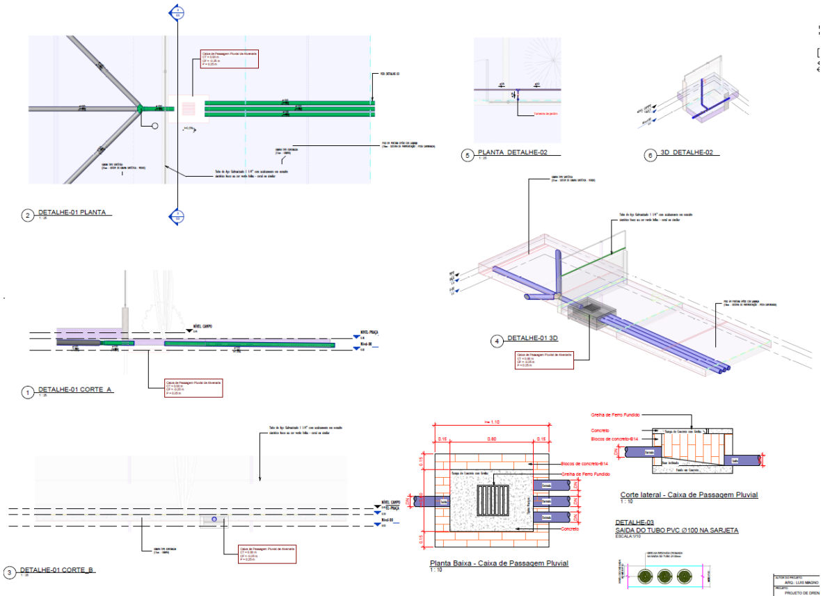
Imagem 09 - Detalhamento do projeto de drenagem
