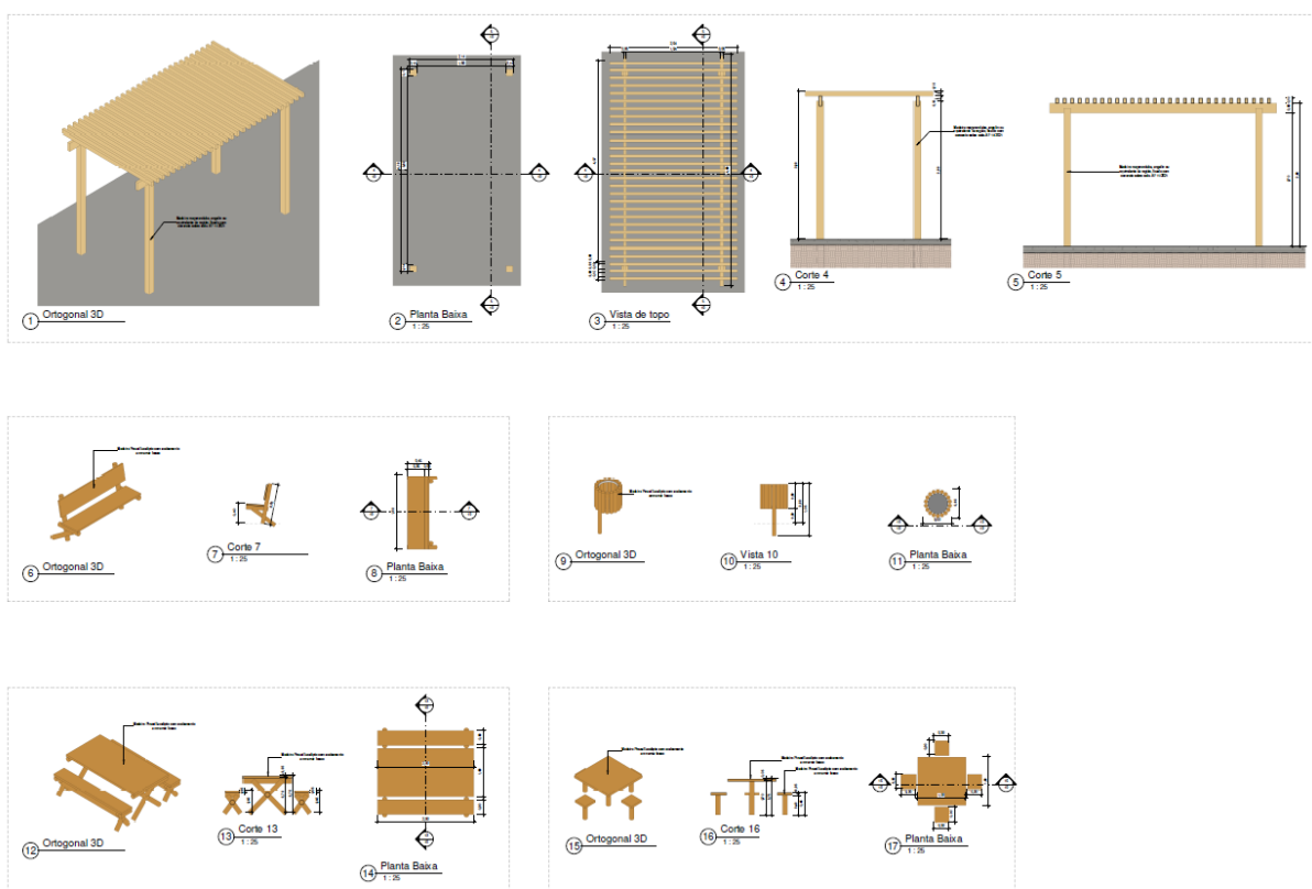
Imagem 05 - Detalhamento do mobiliário
