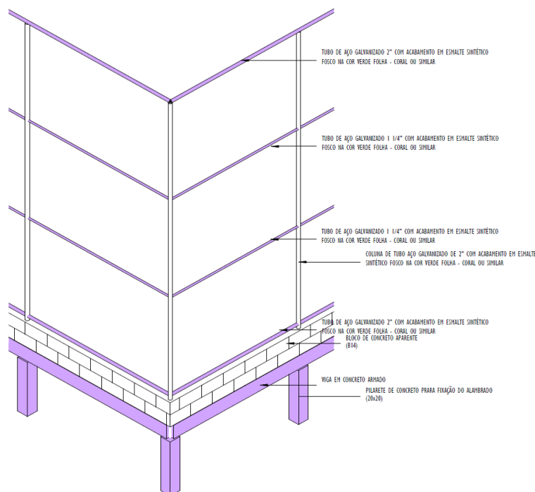
Imagem 04 – Detalhamento do alambrado
