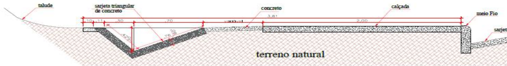
2 Modelo Tipo - Sarjeta de Concreto Triangular - STC02
