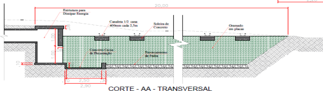
CORTE - AA - TRANSVERSAL esc.: 1 / 500
