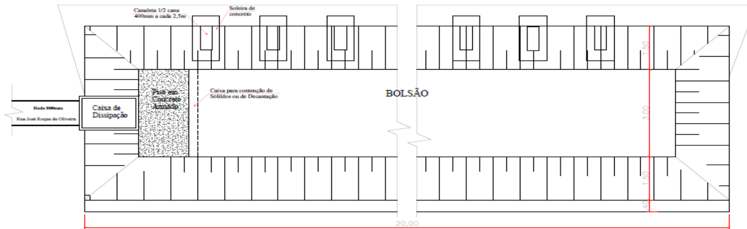
DISSIPADOR DE ENERGIA COM BOLSÃO esc.: 1 / 500
