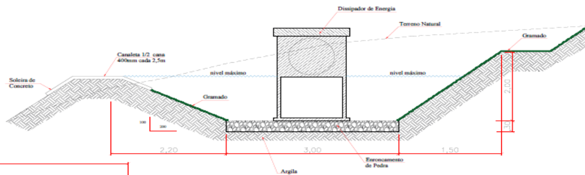
CORTE - BB - LONGITUDINAL esc.: 1 / 500
