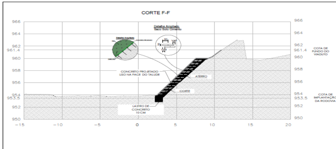
SEÇÃO TRANSVERSAL - CORTE F-F ESCALA 1:100
