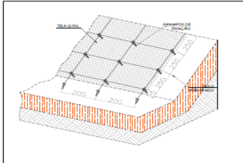
DETALHE INSTALAÇÃO E FIXAÇÃO DA TELA SEM ESCALA
