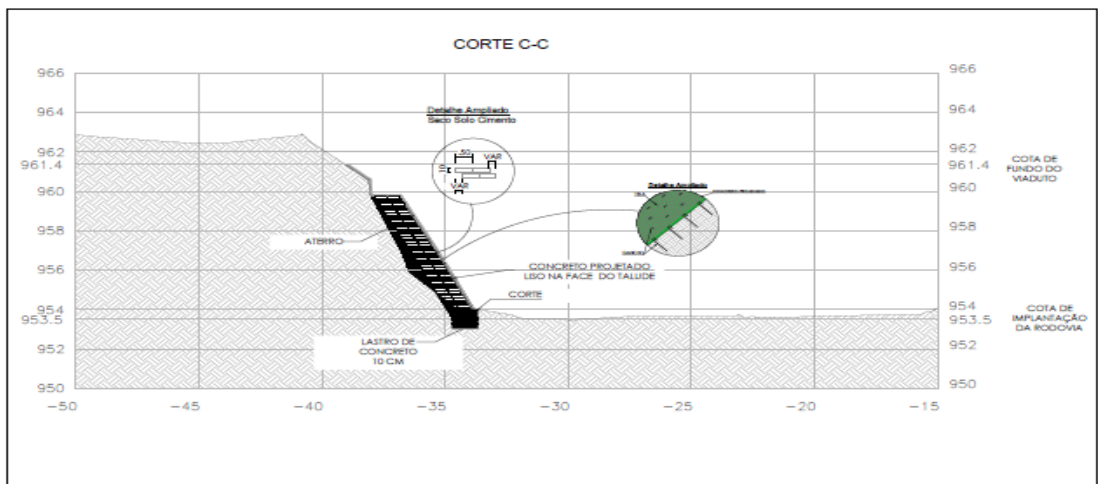
SEÇÃO TRANSVERSAL - CORTE C-C ESCALA 1:100
