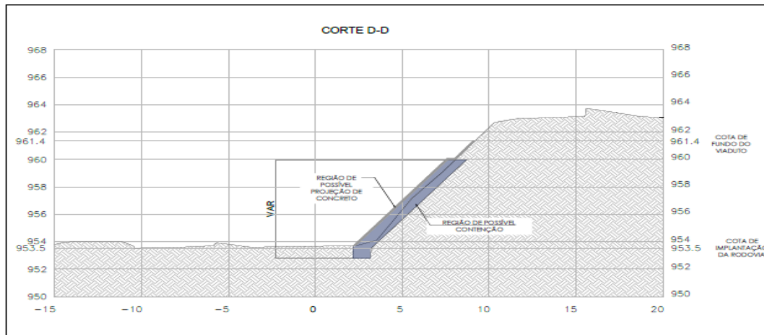
SEÇÃO TRANSVERSAL - CORTE D-D ESCALA 1:100
