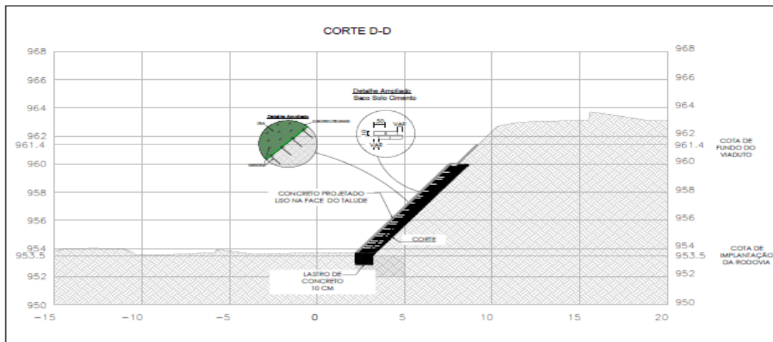
SEÇÃO TRANSVERSAL - CORTE D-D ESCALA 1:100
