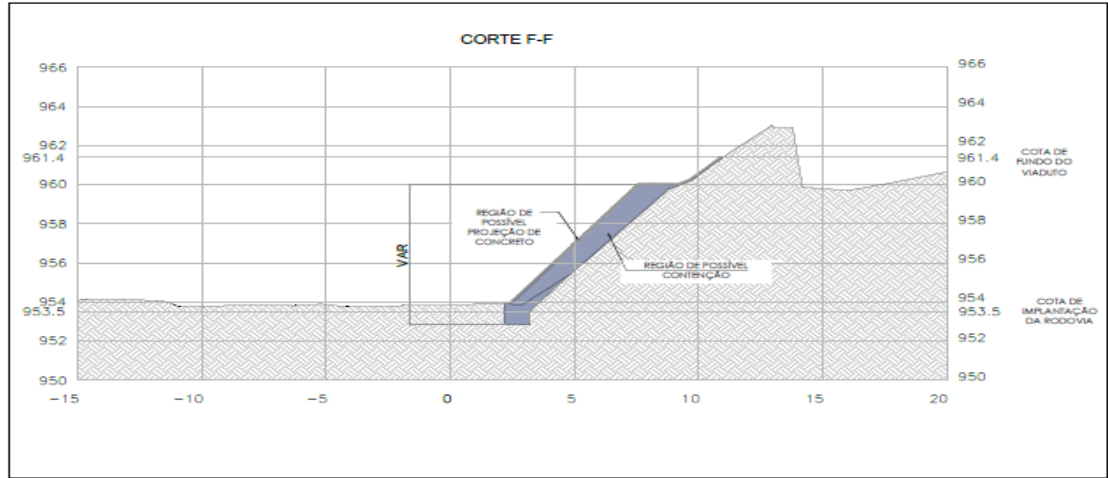
SEÇÃO TRANSVERSAL - CORTE F-F ESCALA 1:100
