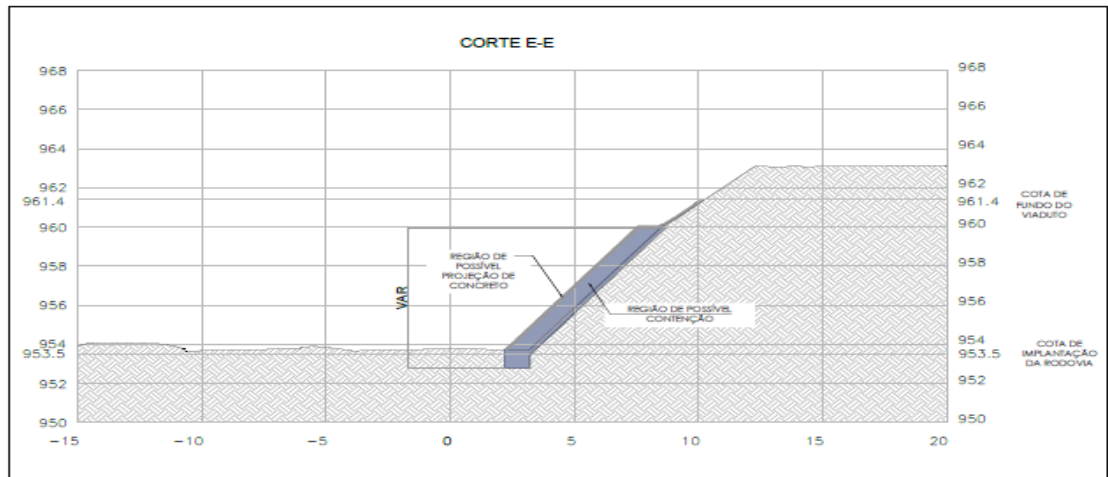
SEÇÃO TRANSVERSAL - CORTE E-E ESCALA 1:100
