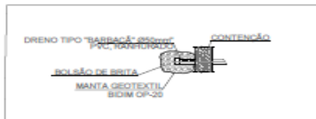
DETALHE - DRENAGEM BARBACA ESCALA 1:50
