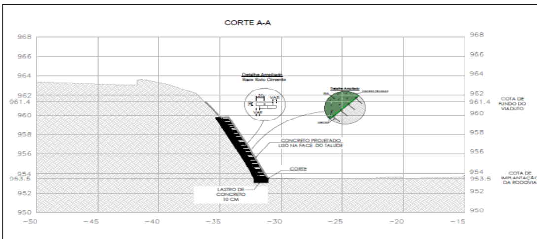
SEÇÃO TRANSVERSAL - CORTE A-A ESCALA 1:100
