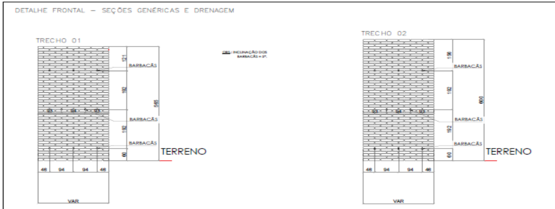
DETALHE FRONTAL - SEÇÕES GÊNICAS E DRENAGEM ESCALA 1:50
