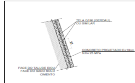
TRASPASSO VERTICAL DA TELA METÁLICA ESCALA 1:25
