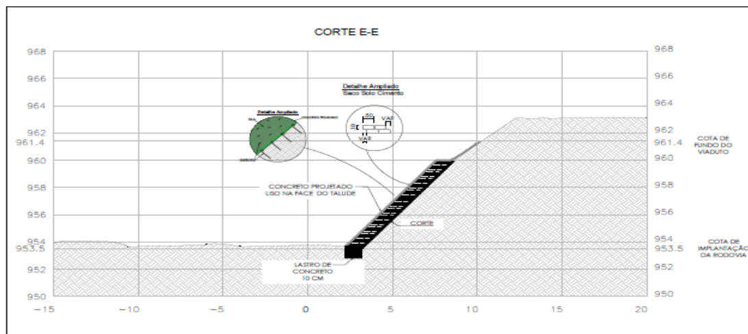
SEÇÃO TRANSVERSAL - CORTE E-E ESCALA 1:100
