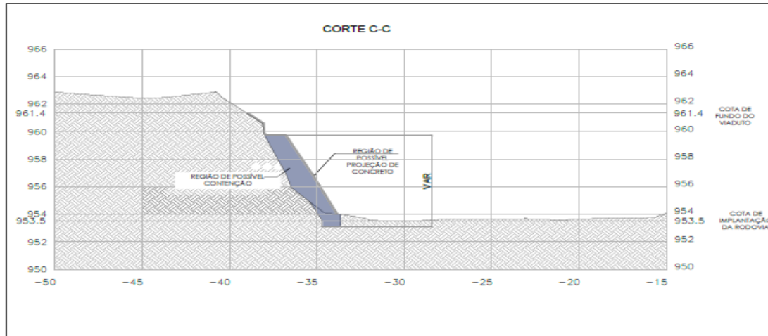
SEÇÃO TRANSVERSAL - CORTE C-C ESCALA 1:100
