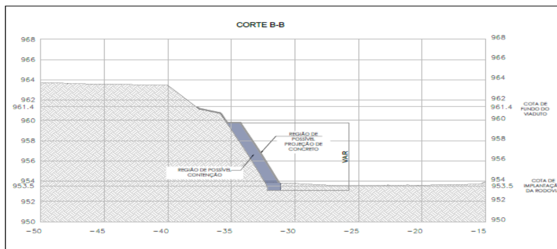
SEÇÃO TRANSVERSAL - CORTE B-B ESCALA 1:100
