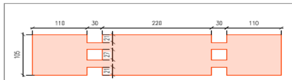
PLANTA DE FORMA - LAJE PRÉ MOLDADA ESCALA 1:25
