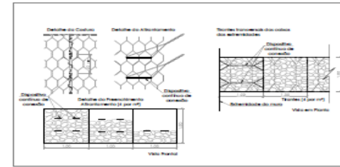
DETALHE TÍPICO - AMARRAÇÃO DA MALHA SEM ESCALA
