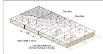
DETALHE TÍPICO - TIRANTES VERTICAIS SEM ESCALA
