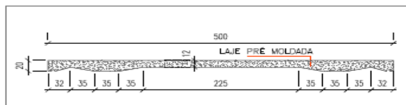
CORTE LONGITUDINAL - LAJE PRÉ MOLDADA ESCALA 1:25
