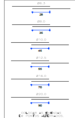
DETALHE DE AMARRAÇÃO DAS BARRAS SEM ESCALA
