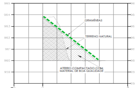
SEÇÃO TRANSVERSAL - CORTE G ESCALA: 1/50
