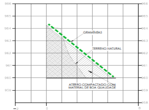
SEÇÃO TRANSVERSAL - CORTE E ESCALA: 1/50
