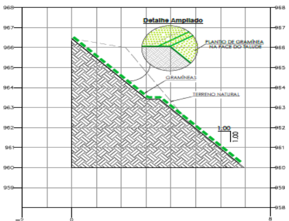
SEÇÃO TRANSVERSAL CORTE A ESCALA: 1/50
