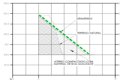
SEÇÃO TRANSVERSAL CORTE G ESCALA: 1/50
