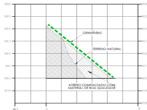
SEÇÃO TRANSVERSAL CORTE F ESCALA: 1/50
