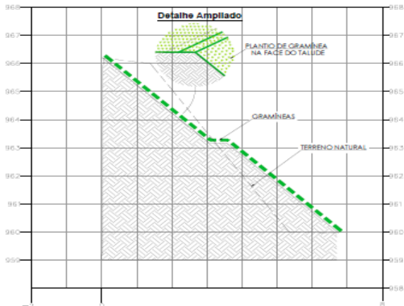
SEÇÃO TRANSVERSAL CORTE D ESCALA: 1/50
