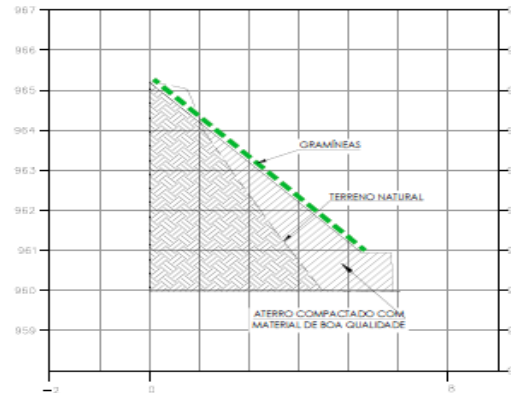
SEÇÃO TRANSVERSAL CORTE E ESCALA: 1/50
