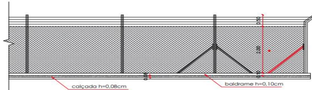
③ DETALHE ALAMBRADO
