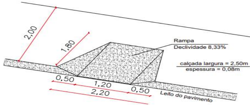
② DETALHE CALÇADA / RAMPA
